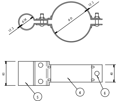
ガードレール取付金具標準詳細図
