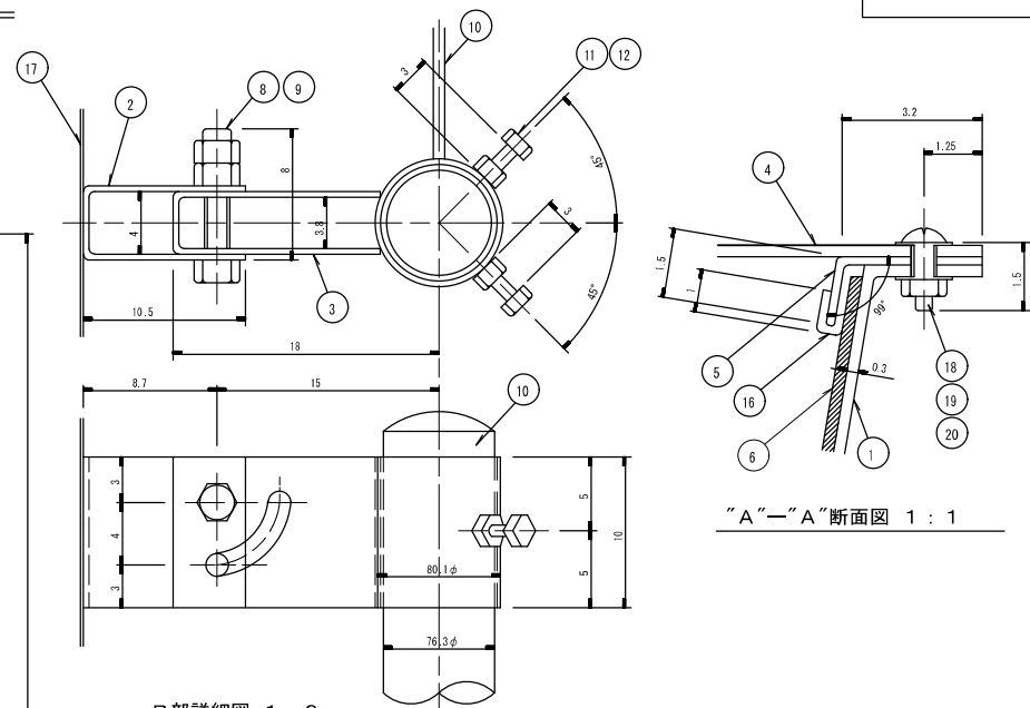
B部詳細図 1 : 3
