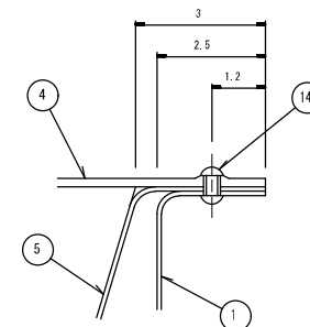
"A"-"A" 断面図 1 : 1
