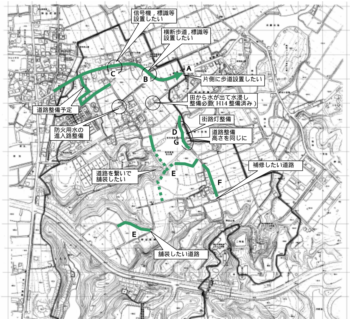
計画図
