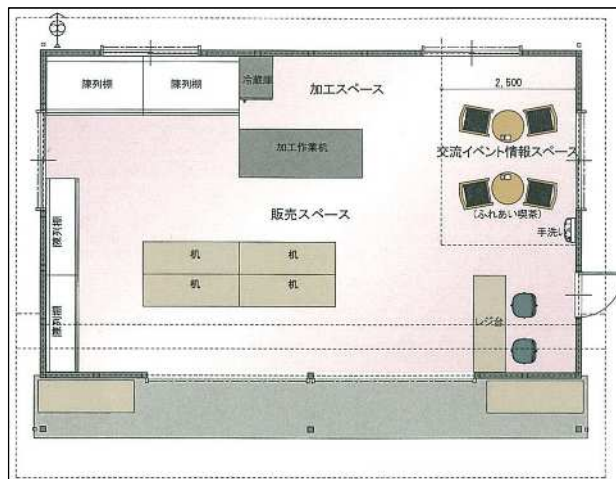
間取り計画図
