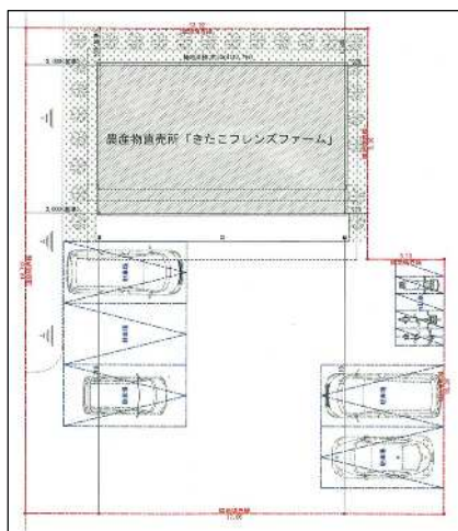
配置計画図
