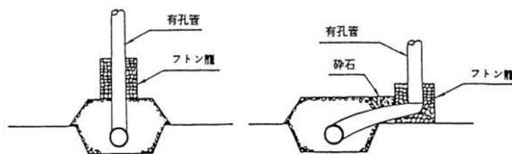
縦型集排水管の例
