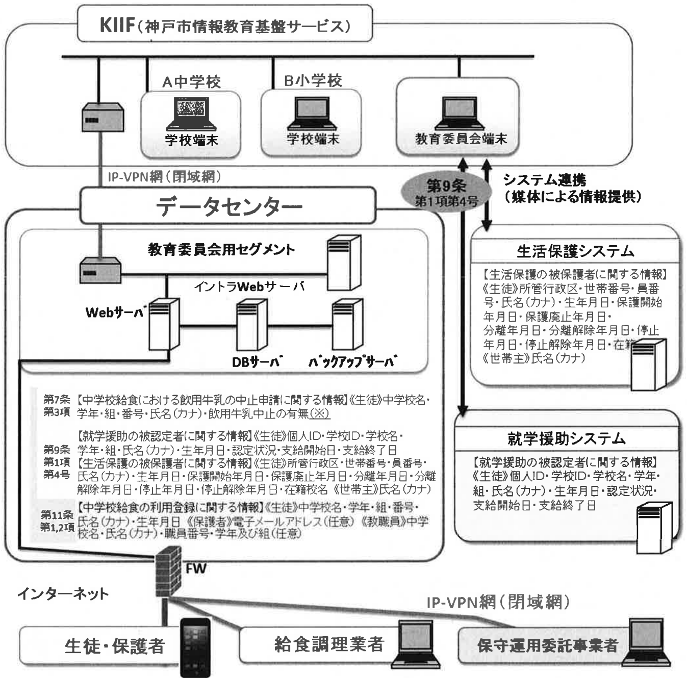
中学校給食予約管理システムの全体図
