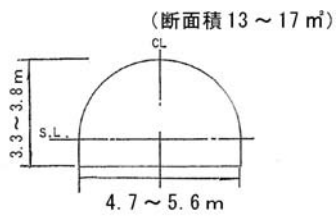
(標準部の断面)
