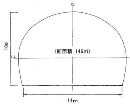
(D3機械室の断面)
