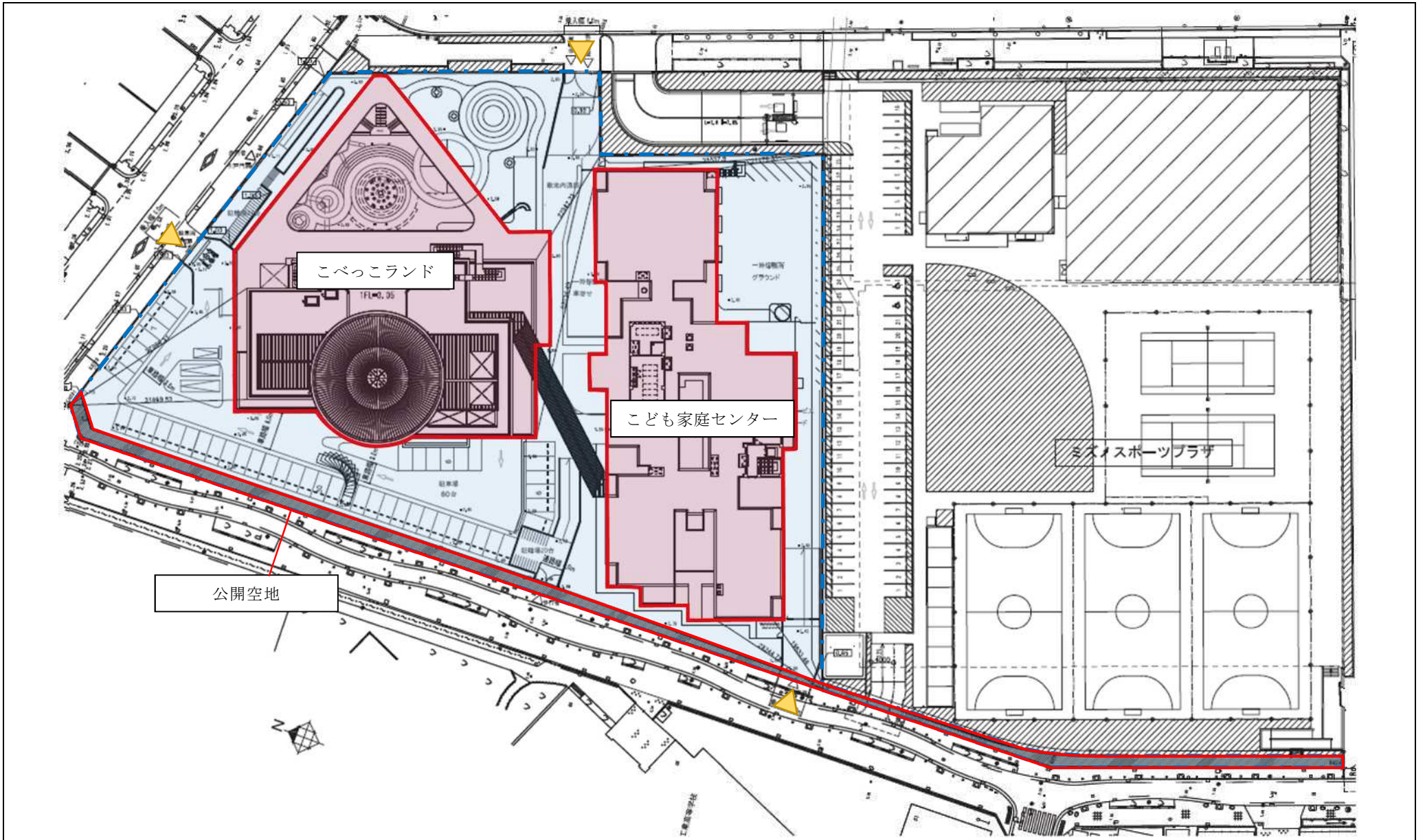
配置図
