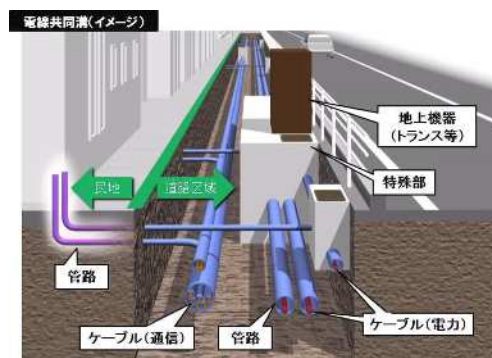
電線共同溝イメージ(出典:国土交通省)
