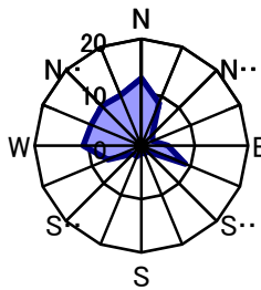
2月 静穏時2.3%
