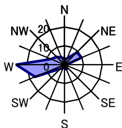
12月 静穏時1.9%
