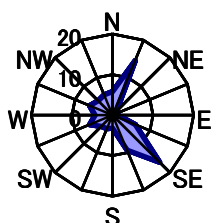
5月 静穏時6.7%
