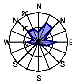
11月 静穏時2.9%
