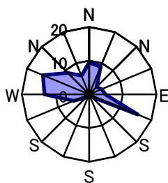
12月 静穏時1.9%
