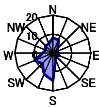
4月 静穏時1.7%
