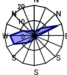
2月 静穏時3.4%
