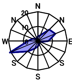
4月 静穏時1.8%
