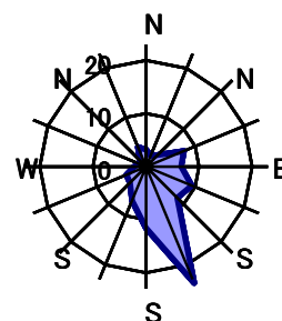
7月 静穏時0.1%
