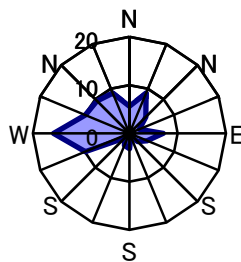
1月 静穏時2.7%
