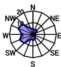
4月 静穏時1.4%
