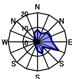
9月 静穏時0.3%
