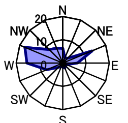
2月 静穏時1.0%
