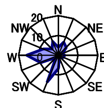
7月 静穏時3.4%
