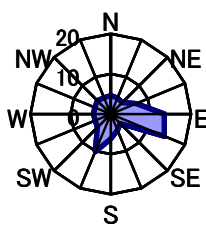
9月 静穏時1.9%
