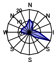
11月 静穏時1.5%
