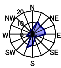
9月 静穏時0.7%
