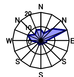
10月 静穏時1.2%
