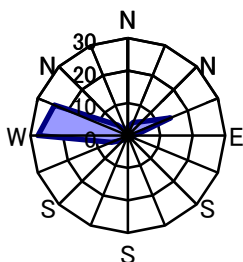
12月 静穏時0.5%
