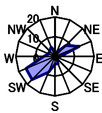
4月 静穏時2.2%
