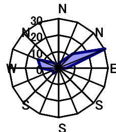
11月 静穏時1.1%
