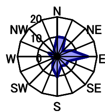
9月 静穏時0.6%
