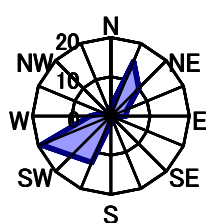
4月 静穏時4.3%
