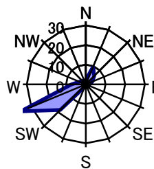
1月 静穏時5.1%
