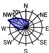
1月 静穏時0.4%
