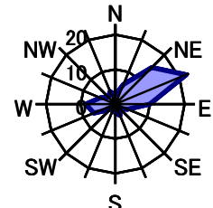
11月 静穏時3.2%
