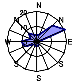
11月 静穏時3.6%
