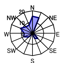
3月 静穏時4.3%
