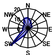
4月 静穏時1.1%
