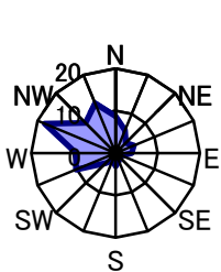
1月 静穏時0.3%
