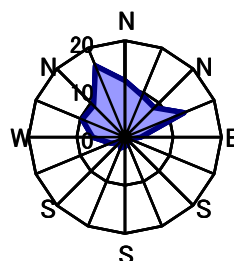
11月 静穏時0.8%
