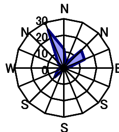
10月 静穏時1.8%
