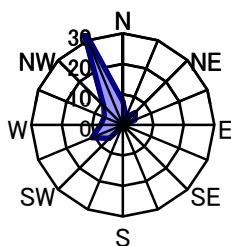
1月 静穏時1.5%
