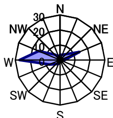
1月 静穏時1.5%
