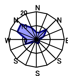
11月 静穏時1.9%
