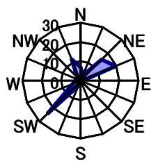
9月 静穏時1.0%
