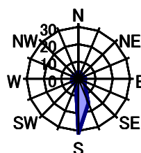
6月 静穏時2.5%
