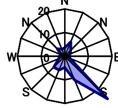
7月 静穏時11.8%
