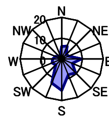
8月 静穏時0.8%
