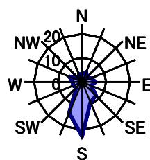
7月 静穏時0.3%
