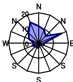
10月 静穏時0.1%
