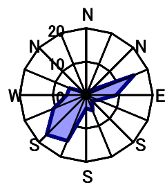
8月 静穏時0.8%
