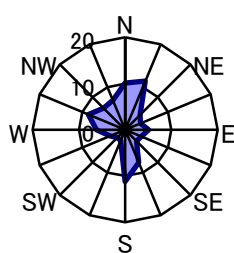
北 静穏時2.0%
