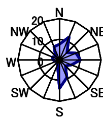
9月 静穏時1.6%
