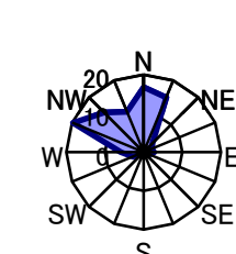
1月 静穏時0.4%
