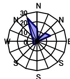
11月 静穏時1.7%
