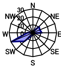
8月 静穏時2.3%
