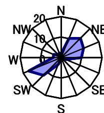
9月 静穏時5.1%
