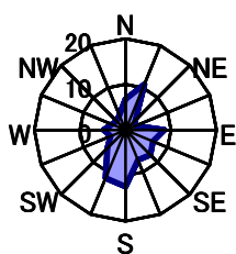
5月 静穏時0.4%
