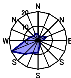
6月 静穏時0.0%
