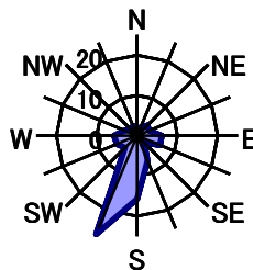
6月 静穏時3.5%
