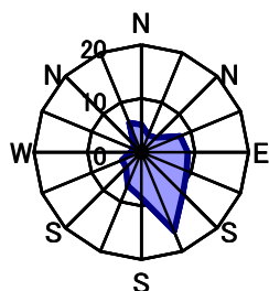
8月 静穏時0.8%
