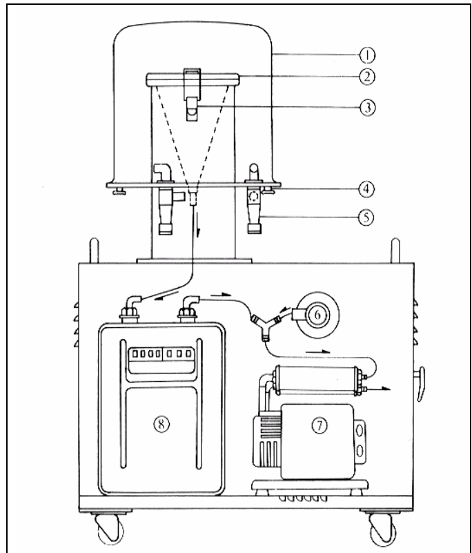
図1 ローボリウムエアサンプラー（新宅FKS型）
