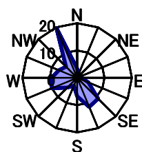
4月 静穏時0.0%
