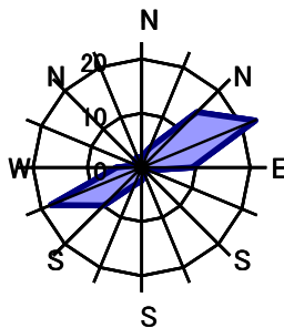
9月 静穏時1.5%
