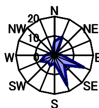
4月 静穏時0.7%
