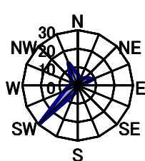
4月 静穏時2.4%
