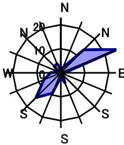
9月 静穏時2.5%
