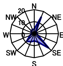
8月 静穏時10.2%
