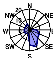
6月 静穏時1.0%
