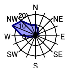
12月 静穏時0.1%
