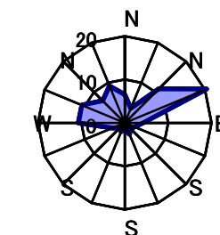
11月 静穏時1.5%
