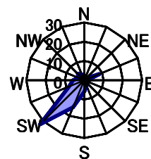
7月 静穏時0.5%
