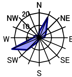
3月 静穏時4.6%
