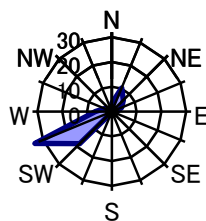
12月 静穏時8.2%
