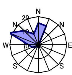
1月 静穏時5.1%
