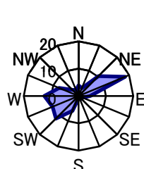
3月 静穏時1.7%
