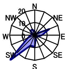
8月 静穏時0.8%
