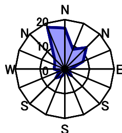
10月 静穏時0.4%
