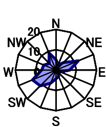
5月 静穏時0.0%
