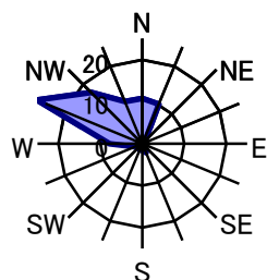
12月 静穏時4.2%
