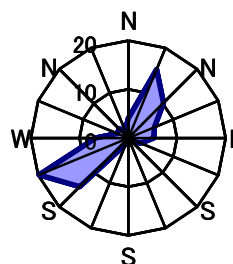
10月 静穏時6.2%
