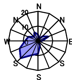
7月 静穏時0.0%
