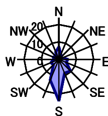
6月 静穏時0.6%
