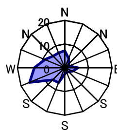
2月 静穏時1.9%
