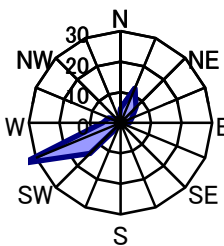
2月 静穏時5.0%
