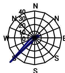
7月 静穏時2.8%
