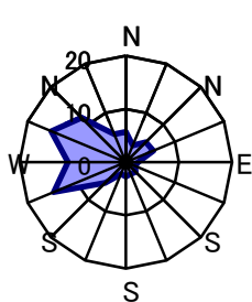
2月 静穏時1.7%
