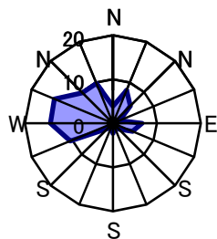
12月 静穏時3.4%
