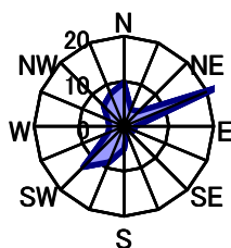
9月 静穏時0.6%
