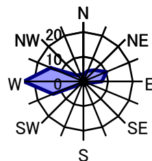
12月 静穏時2.0%
