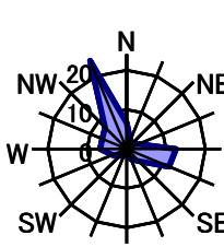
10月 静穏時0.5%
