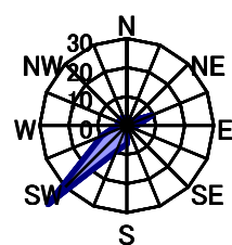
6月 静穏時1.0%
