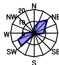
8月 静穏時3.2%
