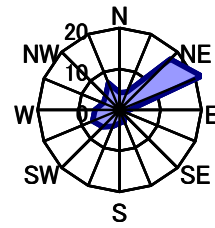
10月 静穏時2.3%
