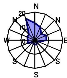
11月 静穏時0.1%
