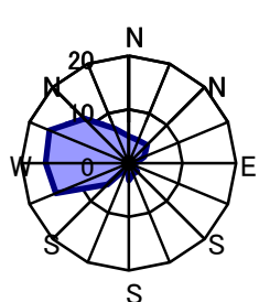
1月 静穏時1.7%
