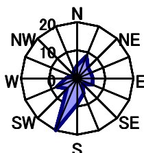
5月 静穏時3.8%
