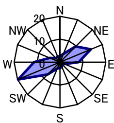
葦合 静穏時1.3%
