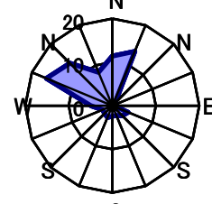
11月 静穏時10.1%
