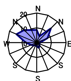
10月 静穏時0.9%
