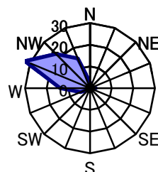
12月 静穏時0.1%
