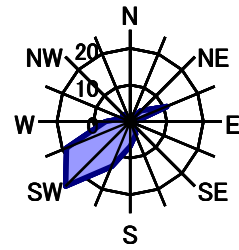
7月 静穏時0.8%
