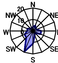
6月 静穏時1.9%
