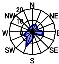
5月 静穏時1.6%
