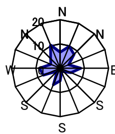
3月 静穏時4.3%
