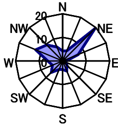
9月 静穏時1.4%
