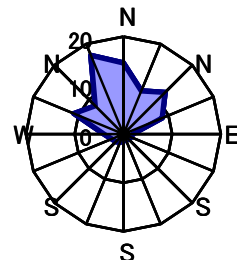
11月 静穏時0.3%
