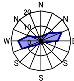
2月 静穏時2.4%
