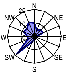
須磨 静穏時1.1%
