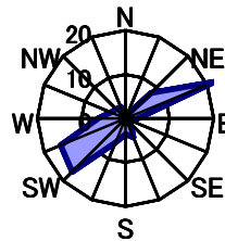
5月 静穏時1.1%
