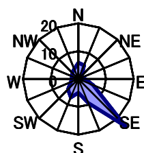
6月 静穏時13.6%
