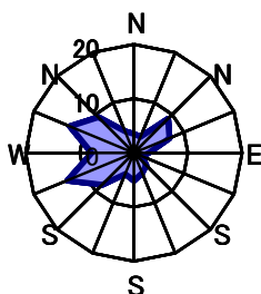
5月 静穏時0.7%
