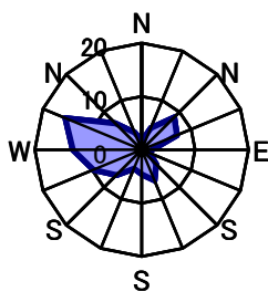
8月 静穏時1.2%
