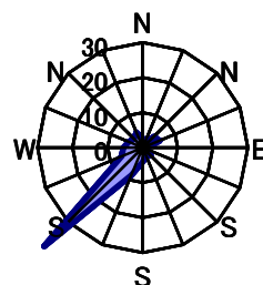
7月 静穏時1.6%
