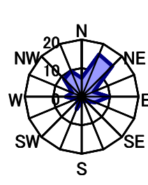
10月 静穏時3.2%
