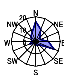
10月 静穏時0.8%
