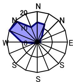
12月 静穏時1.6%
