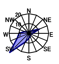
6月 静穏時0.8%
