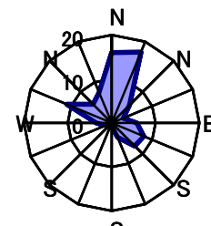
11月 静穏時1.5%
