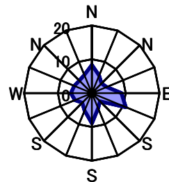
10月 静穏時2.8%
