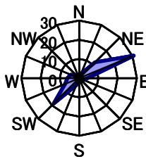
9月 静穏時1.5%
