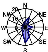
5月 静穏時2.3%
