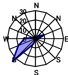
7月 静穏時1.1%
