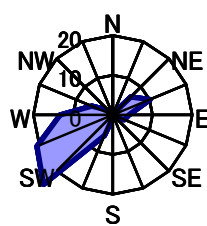
6月 静穏時1.9%
