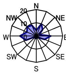
2月 静穏時4.2%
