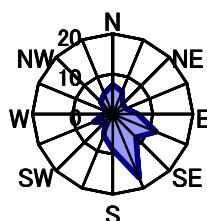
5月 静穏時0.9%
