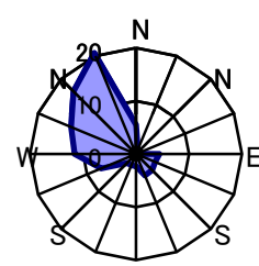
3月 静穏時0.1%
