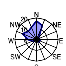
2月 静穏時0.4%
