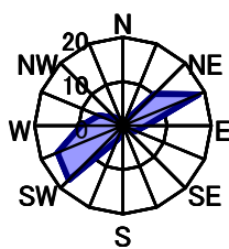
5月 静穏時2.2%
