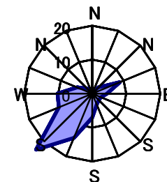
7月 静穏時0.9%
