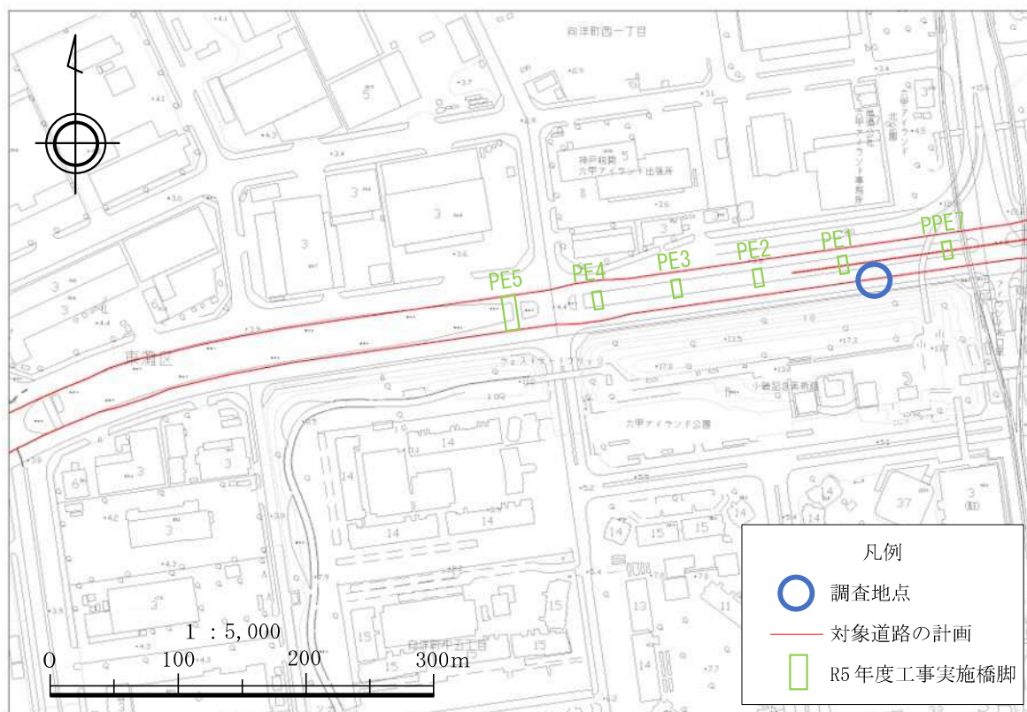
図 5-8 調査位置詳細図（東灘区向洋町中 5 丁目）
