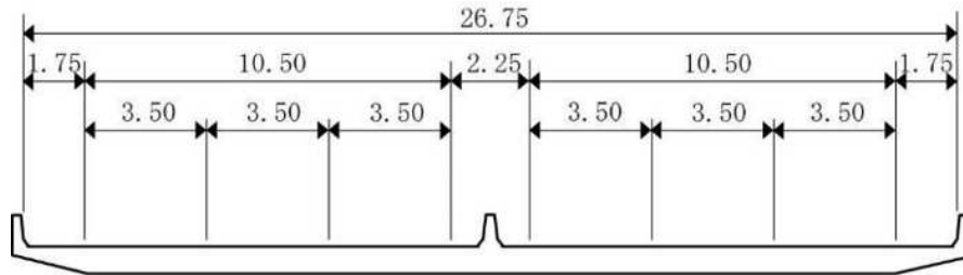
図 2-4 標準断面図
