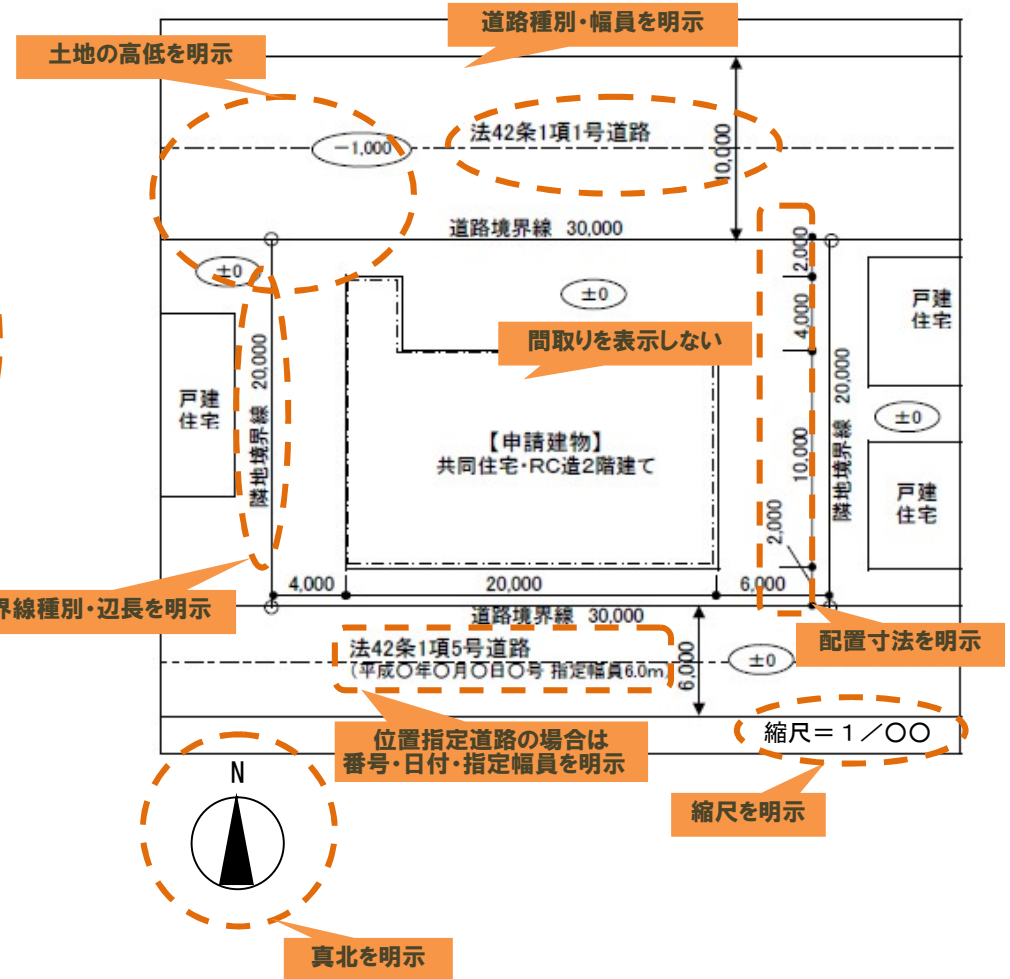
配置図
